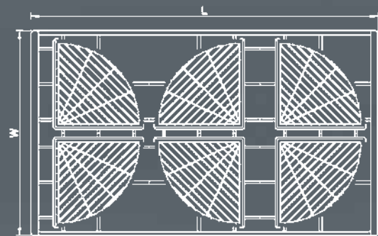
Κάτοψη καλούπιου βαρελιού Layout of block mould for barrel
